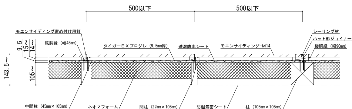
水平断面图
